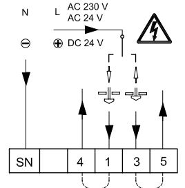
AMV 335, AMV 435
